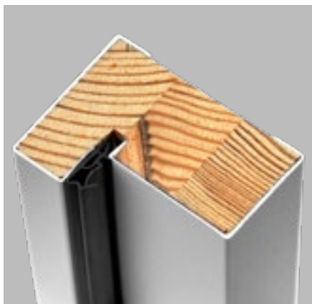
PRIEREZ RÁMU
