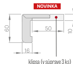
klipsa (v súprave 3 ks)
