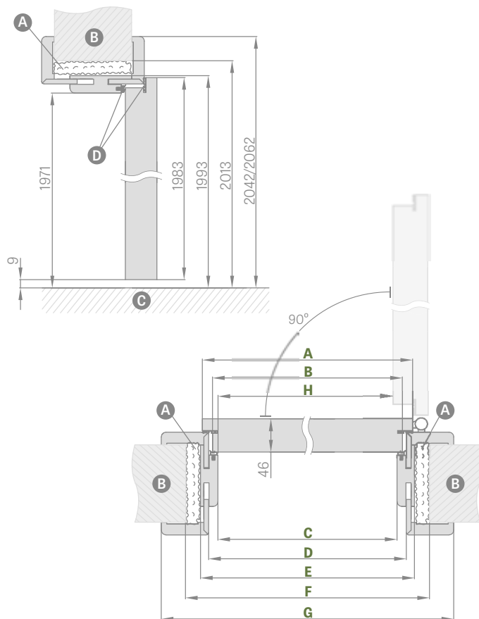
SCHÉMA NASTAVITEĽNEJ ZÁRUBNE HERSE SET
