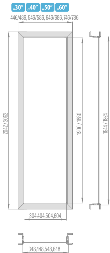
Bočné svetlíky nastaviteľnej zárubne, 6 cm obložka / 8 cm obložka
