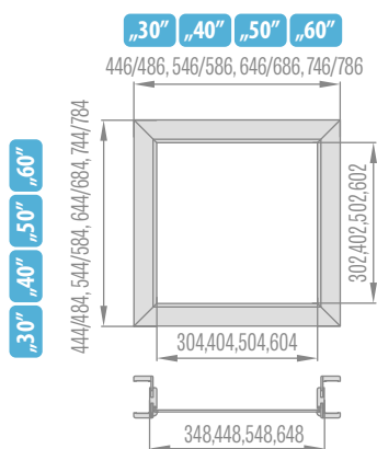
Horné svetlíky s nastaviteľnej dvojkrídlovej zárubne, 6 cm obložka / 8 cm obložka
