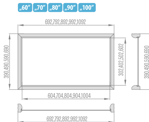
Horné svetlíky pevnej jednokridlovej zárubne
