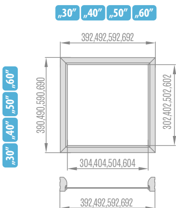
Rohové svetlíky pevnej zárubne
