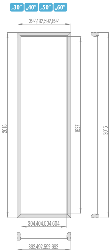
Bočné svetlíky pevnej zárubne
