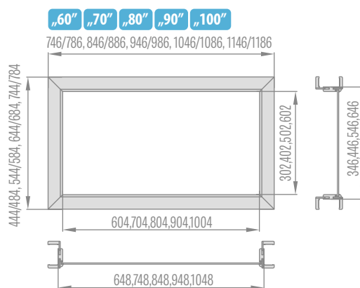
Horné svetlíky nastaviteľnej jednokridlovej zárubne, 6 cm obložka / 8 cm obložka
