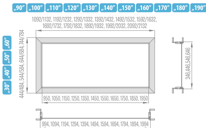
Horné svetlíky s nastaviteľnej dvojkrídlovej zárubne, 6 cm obložka / 8 cm obložka
