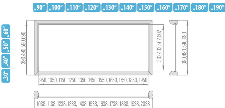
Horné svetlíky pevnej dvojkrídlovej zárubne
